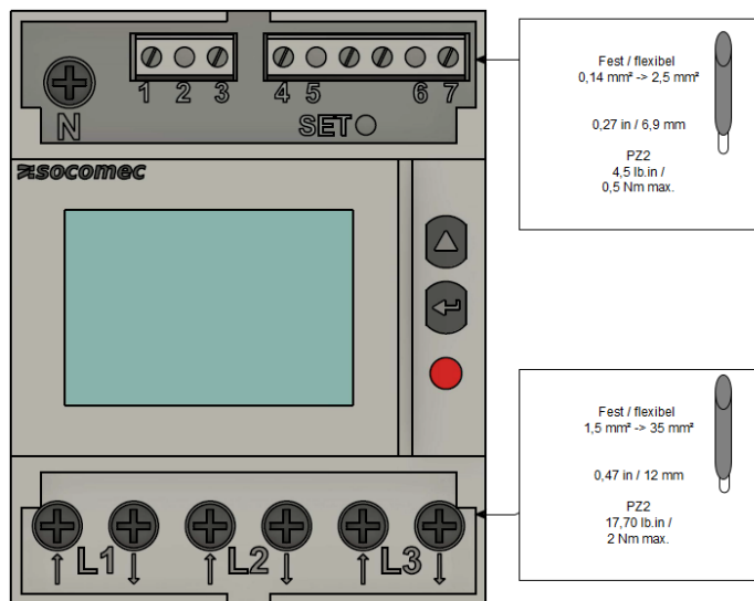
Abbildung 1. Verschraubung
